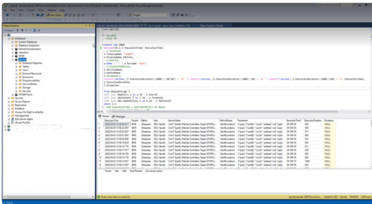
Code Updates
